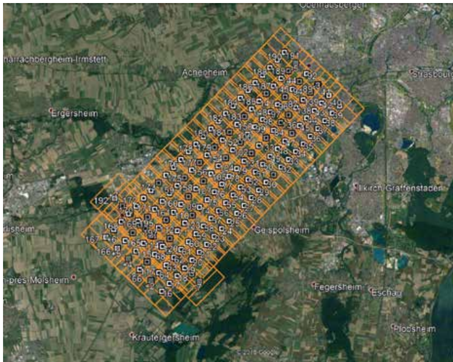
Figure 3. Exemple de plan de vol sur l'aéroport de Strasbourg.
